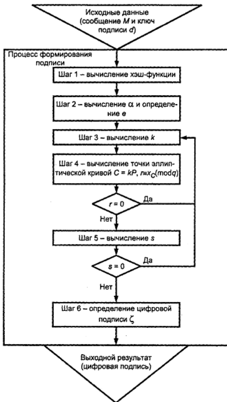
Рисунок 2 - Схема процесса формирования цифровой подписи
