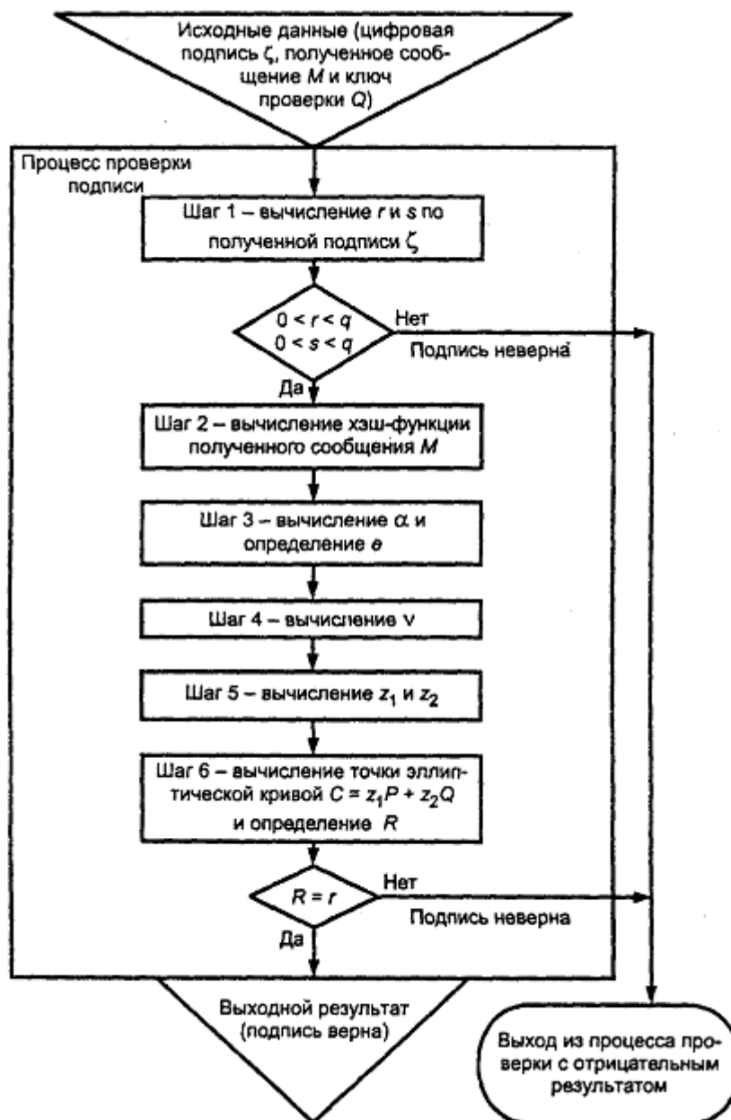
Рисунок 3 - Схема процесса проверки цифровой подписи
